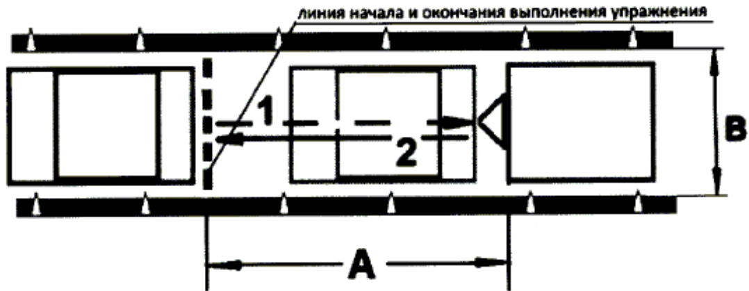
Рисунок 14. Схема и размеры элемента упражнения N 9 - "Сцепление прицепа с тягачом"
