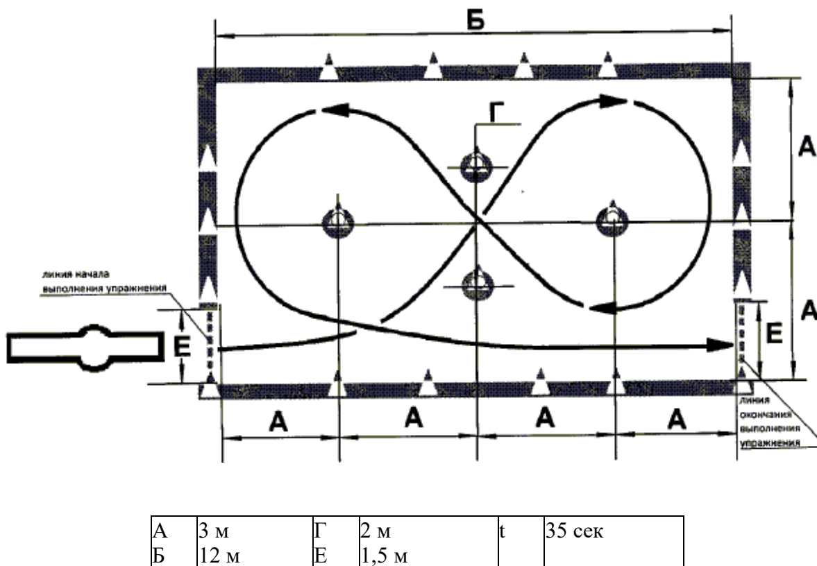
Рисунок 1. Схема и размеры элемента упражнения N 1 - "Габаритная восьмерка"
